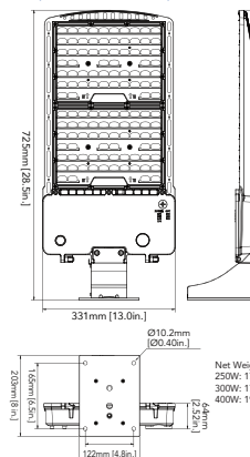
300W/400W (Wall Mount)
