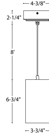
Pendant Cable-mount
