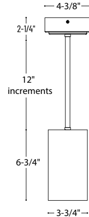
Pendant Stem-mount
